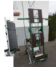
Cadre pour panneaux solaires : pour le transport vertical des panneaux solaires et photovoltaïques de taille variable.
